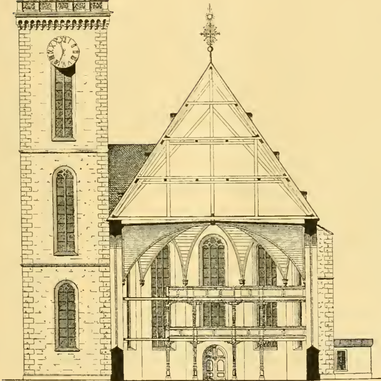
Fig. 16. Katharinenkirche zu Frankfurt a. M. Querschnitt.
